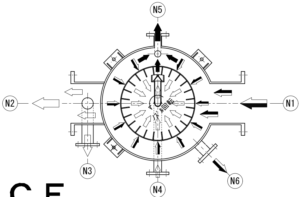
DCF型オートストレーナ 濾過・逆洗 流路図
